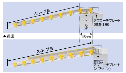
▲耐荷式アプローチプレート(オプション)の使用例
